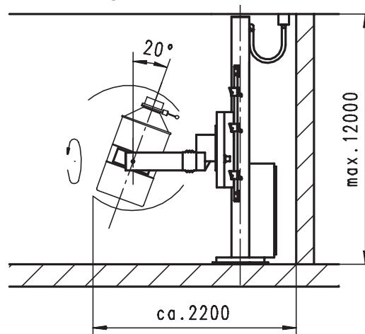
Mélangeur de fût avec fonction de levage
