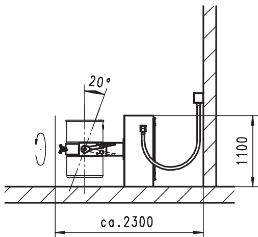
Mélangeur de fût sans fonction de levage
