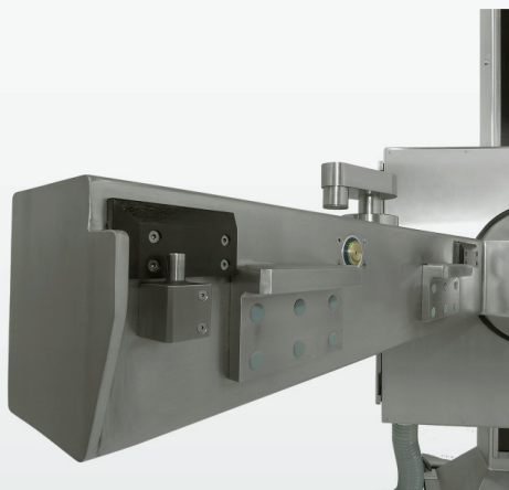
Blocage automatisé par deux vérins de blocage pivotants et deux vérins de centrage latéraux
