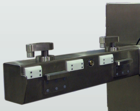
Blocage automatisé par quatre vérins de blocage pivotants et deux vérins de centrage latéraux
